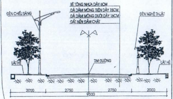
MẶT CẮT NGANG ĐIỂN HÌNH MẶT ĐƯỜNG
